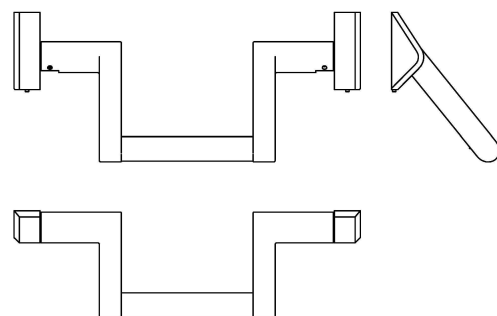
BKS B 74020-00-0-8 Griffrohr
