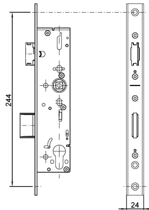
mit Falle und Riegel
