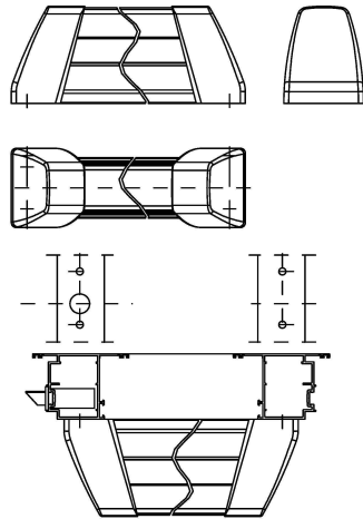
Panikdruckstange (Push bar) (dreiteilig) CE-Z: 0432-CPD-002
