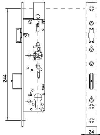
mit Falle und Riegel und oberer Verriegelung
