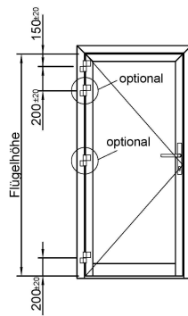
2-teiliges Türband Serie: Dr. Hahn 60AT
