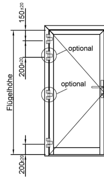
3-teiliges Türband Serie: Dr. Hahn 60AT
