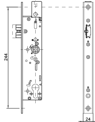
mit Fallenriegel und oberer Verriegelung
